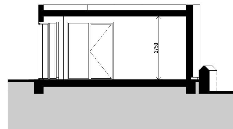
DOORSNEDE B-B
