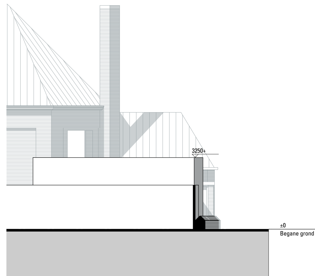
ZIJGEVEL (RECHTS)
