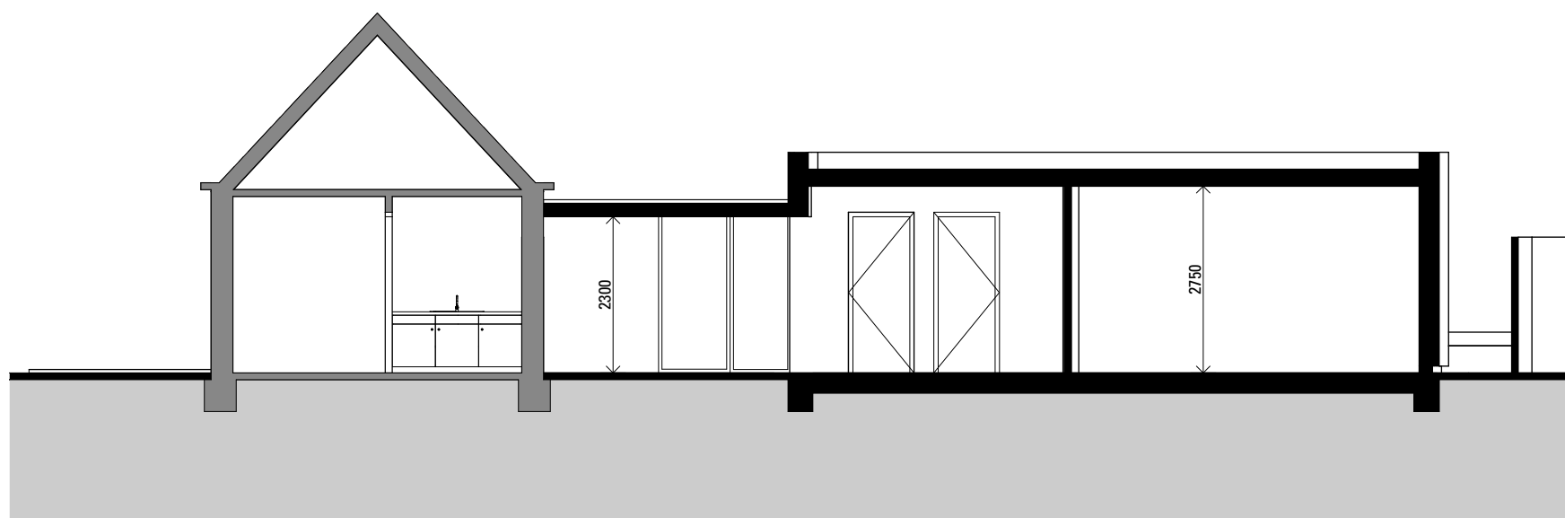
DOORSNEDE A-A
